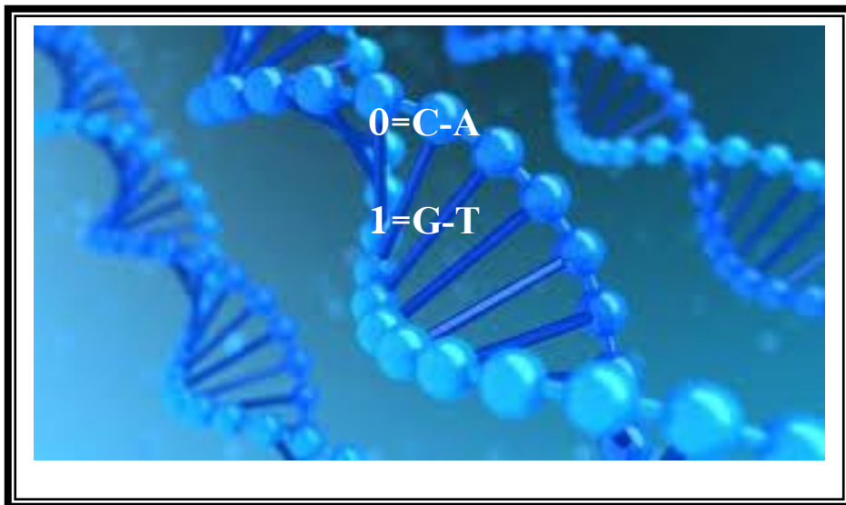
شكل 3: الطريقة الثانية لتشفير البيانات على الحمض النووي DNA.
